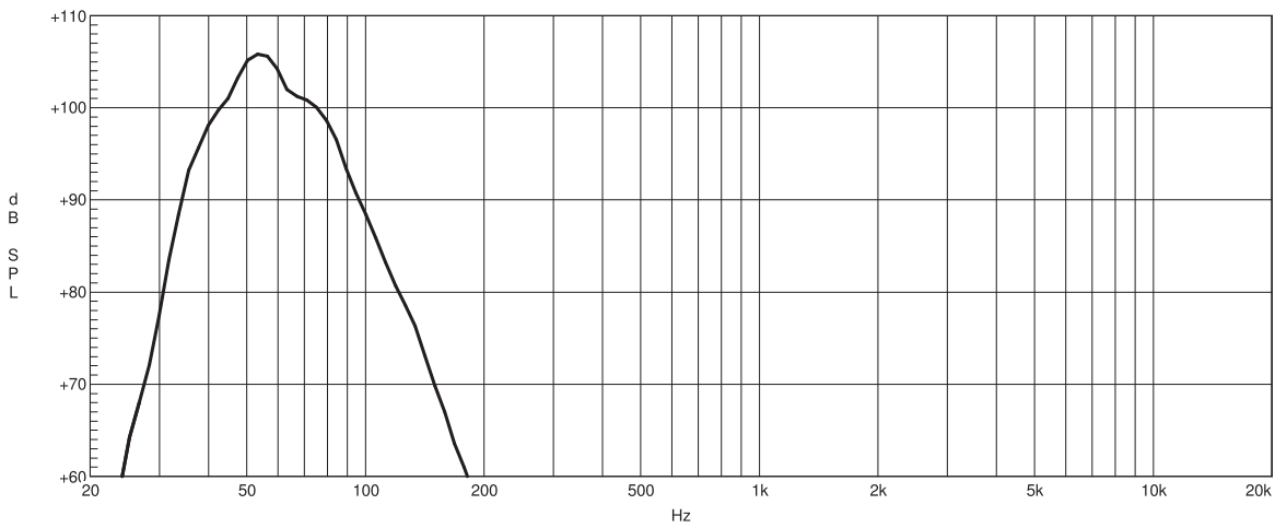
APX 18SA
