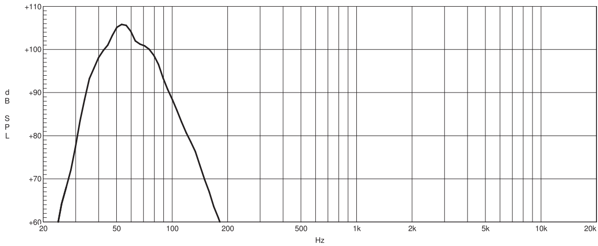
APX 18SA
